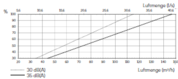
Kapazität mit ePM 10 50% + ePM 10 50% filtern 1
