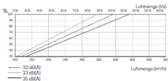
Kapazität mit EPM 1 80% / EPM 10 50% Filter 1
